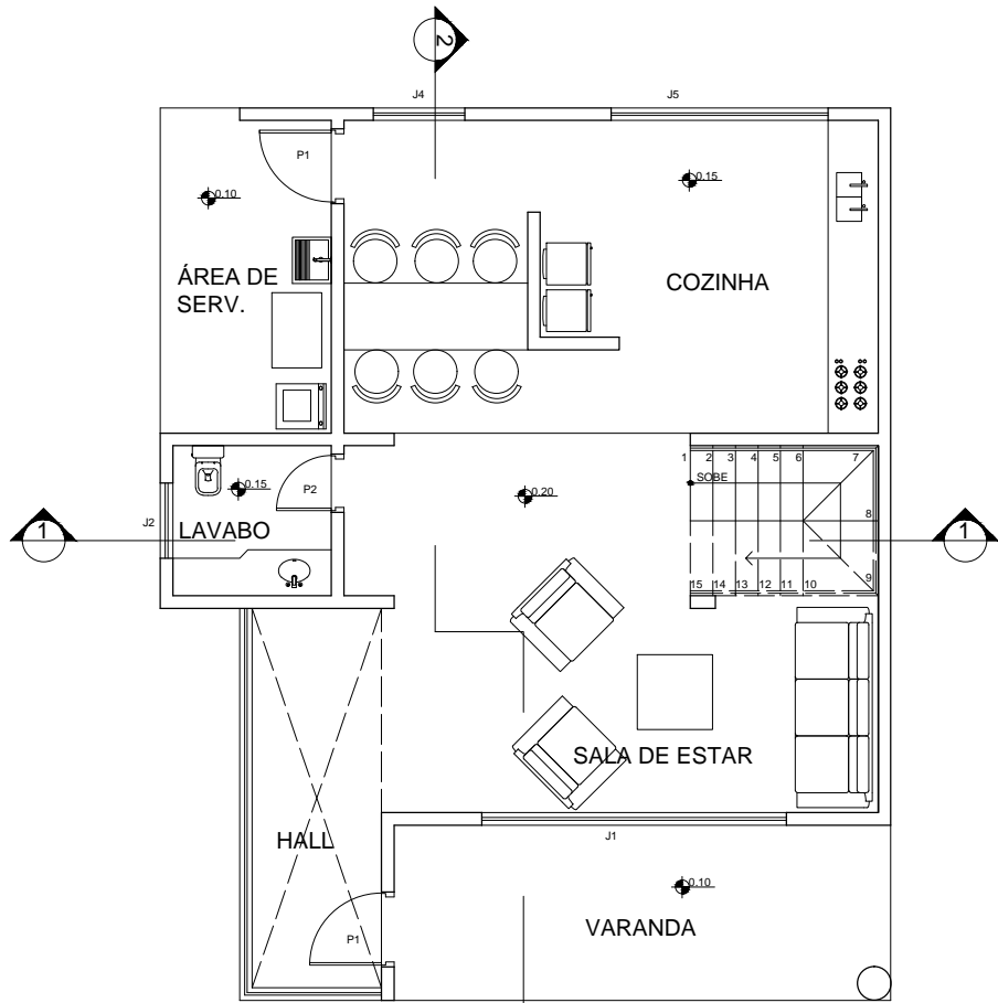
PLANTA PAV. TÉRREO ESC. 1/100
