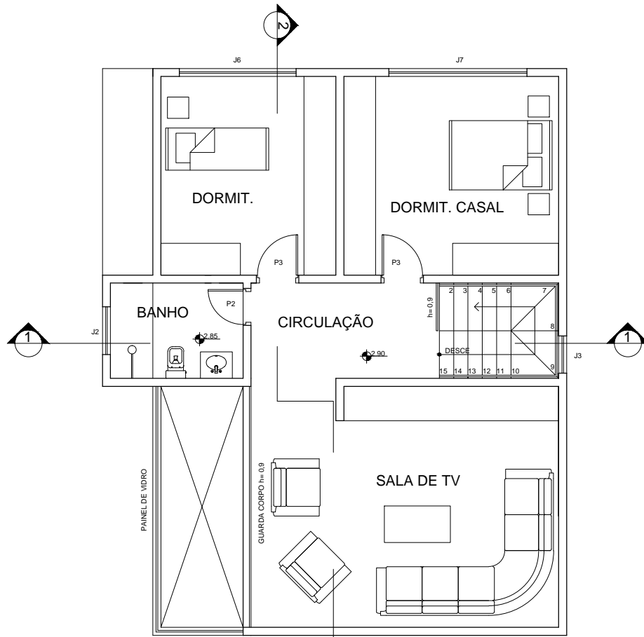
PLANTA PAV. SUPERIOR ESC. 1/100
